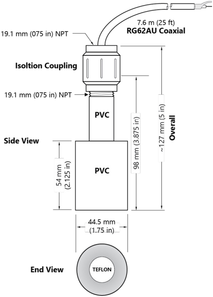
PZ32T sensor
