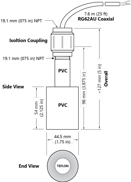
PZ32T sensor
