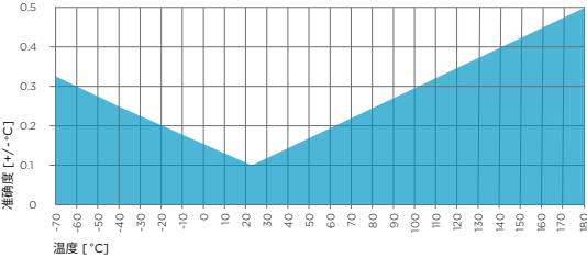
满量程上的 TMP1 温度测量准确度
