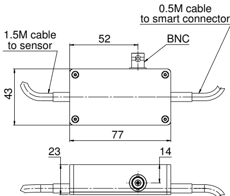
Interface Module
