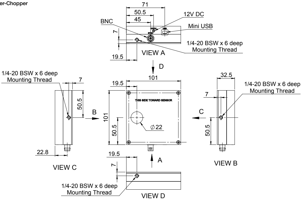
Radiometer-Chopper
