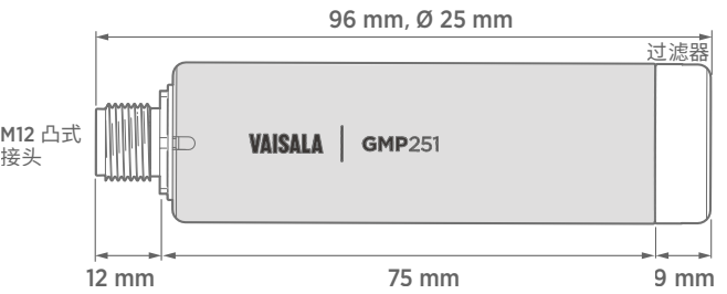
GMP251 尺寸
