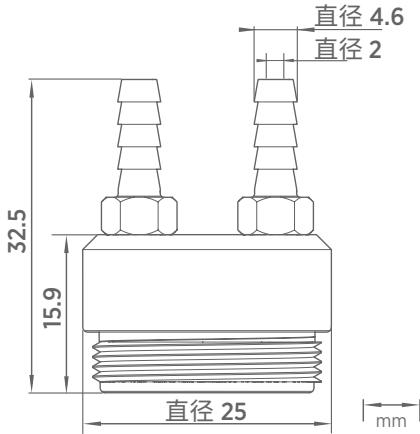
配备气口的流通式适配器。适用于内径为 4 mm 的管。
